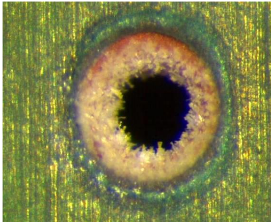
Abb. 5: auskristallisierte Flüssigkeitsrückstände
